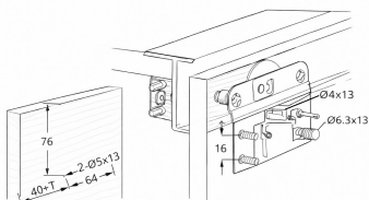
4 Accesorio parte posterior puerta parte superior Top runner rear door
