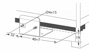
7 Accesorio parte frontal puerta parte inferior Bottom runner front door
