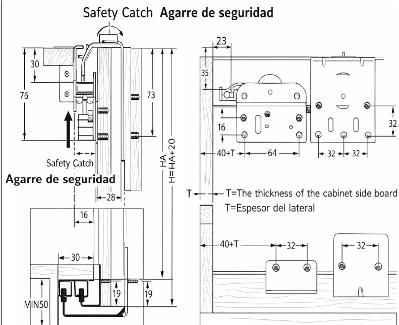
5 Accesorio parte frontal puerta parte superior Top runner front door
