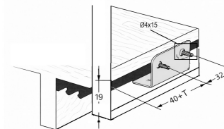
6 Accesorio parte posterior puerta parte inferior Bottom runner rear door
