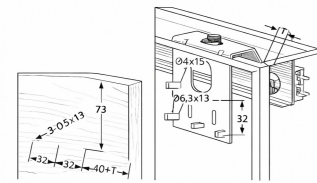
5 Accesorio parte frontal puerta parte superior Top runner front door
